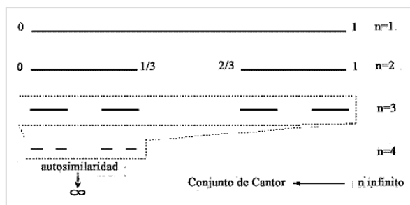
Figura 2. Conjunto de Cantor.
