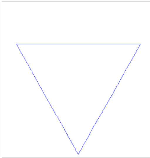
Figura 1. Esquema fractal triangular.
