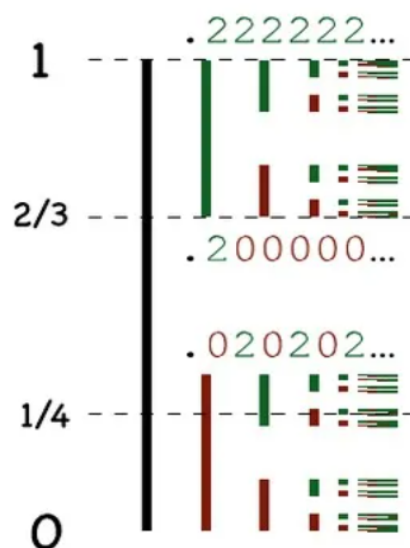
De izquierda a derecha, sucesivos pasos de la construcción geométrica del conjunto de Cantor. Para ilustrar la definición numérica se destacan cuatro puntos del conjunto (0, 2/3, 1 y 1/4) y su expresión en base 3.
